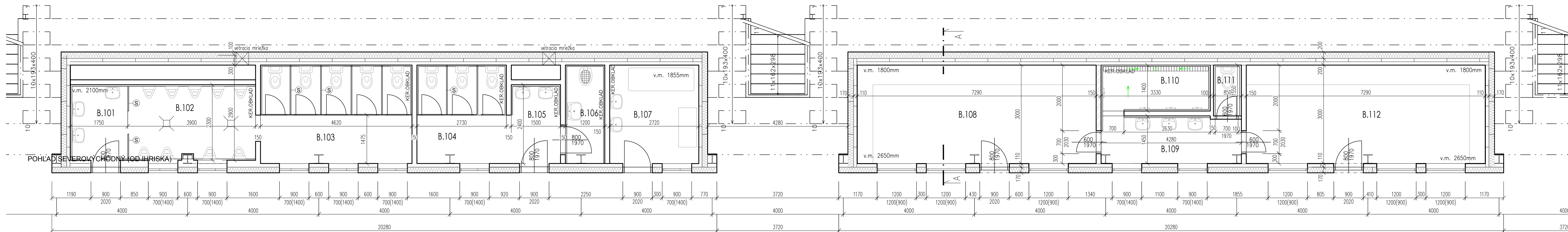
PÓDORYS 1 NP SO 002.B - ČASŤ 2
